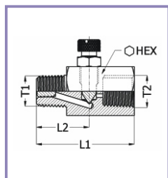
中止開關 On/Off Valve
